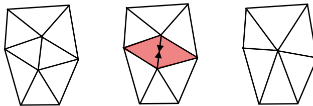
FIGURE 140. Edge collapsing
